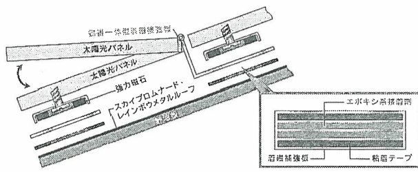
▲新工法は磁石でパネルを取り付ける
